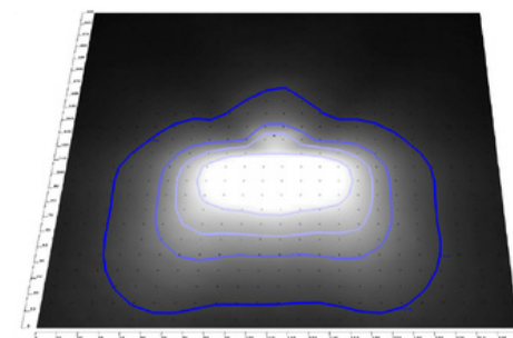
LFXMAX-LG-LENS-TFTM LFXMAX-LG TYPE TFTM LENS
