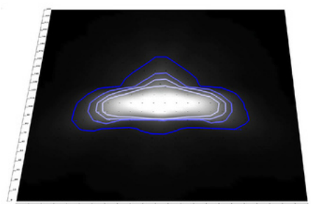
LFXMAX-LG-LENS-T1S LFXMAX-LG TYPE T1S LENS
