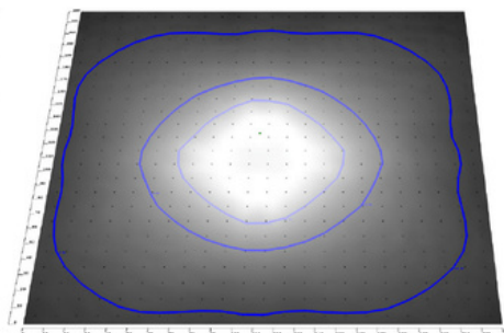
LFXMAX-LG-LENS-T5W LFXMAX-LG TYPE T5W LENS
