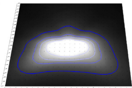
LFXMAX-LG-LENS-T4M LFXMAX-LG TYPE T4M LENS
